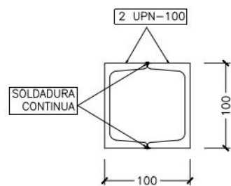
DETALLE DE PUNTALES SUPERIORES
