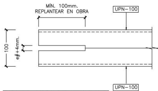
DETALLE DE REBAJE EN PUNTALES PARA UNIÓN CON ARCADAS
