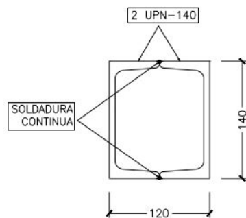
DETALLE DE DIAGONALES
