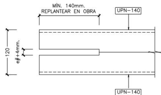
DETALLE DE REBAJE EN DIAGONALES PARA UNIÓN CON ARCADAS
